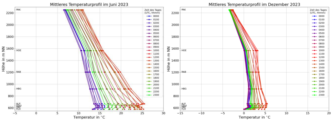
Abbildung A7: Monatsmittel der stündlichen Temperaturprofile im Juni (links) und Dezember (rechts) im Jahr 2023. Die Skala reicht im Juni von -5 bis +30 °C, im Dezember ist sie um 10 °C nach links verschoben. Zur Umrechnung auf Mitteleuropäische Zeit (MEZ) ist eine Stunde zu addieren, 12 Uhr UTC entspricht also beispielsweise 13 Uhr MEZ.
